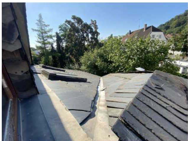
Rückwärtiger Dachbereich, Detail Kehle, Fehlstellen / Bruchstellen / Reparaturen
